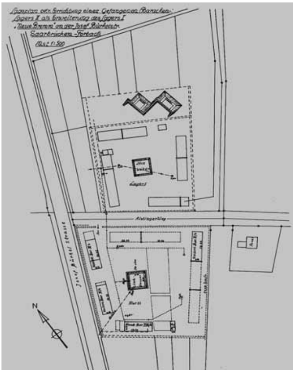
Bauplan zur Errichtung des Gestapo-Lagers Neu-Bremm, Dezember 1943
