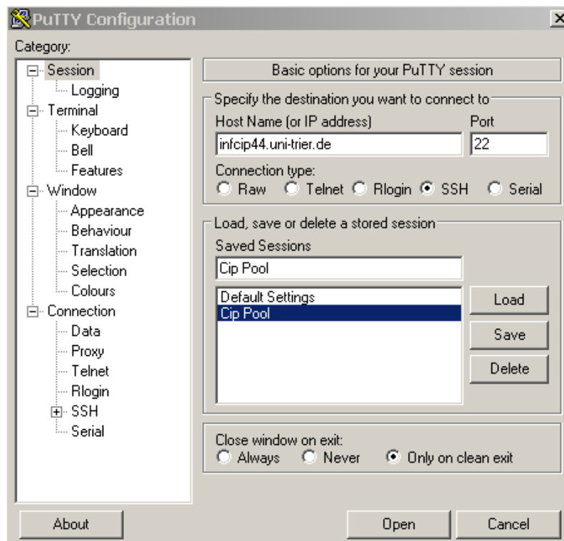
Abbildung 4: PuTTY Eingaben
